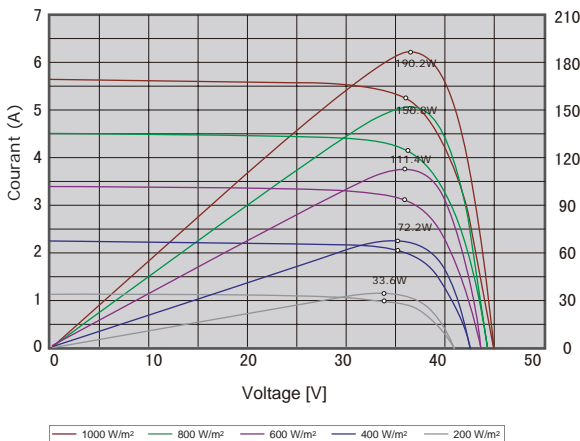
Performance électrique (température des cellules : 25°C)
